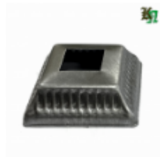
Основание баясины, арт. 8.6020 60x60x1мм, кв.20x20мм Вес: 0.04 кг Цена (за шт): 43 руб.
