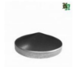
Заглушка, арт. 16.114.01 д=114x1мм Вес: 0.112 кг Цена: 50 руб.
