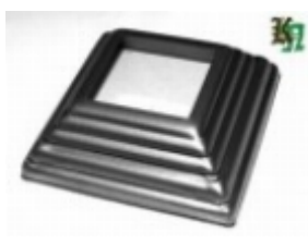
Основание блясины, арт. 13.350.01 100x100x1мм, кв.50x50мм Вес: 0.064 кг Цена: 37 руб.
