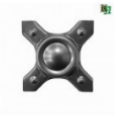
Декоративный колпачок, арт. 1911.36 65x65мм, д=35мм, под трубу 10x10мм Вес: 0.02 кг Цена: 19 руб.
