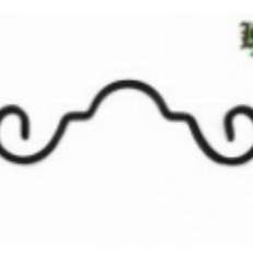
Элемент орнамента - вензель, арт. 19025 250x75мм, полоса 6x12мм Вес: 0.24 кг Цена: 90 руб.
