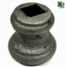
Вставка в балясину, арт. 13.163 50x47мм, на кв.16x16мм Вес: 0.23 кг Цена (за шт): 60 руб.
