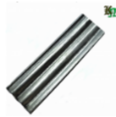
Обжимка, арт. 015201 1250x15x1,5мм Вес: 0.14 кг Цена (за штуку): 43 руб.
