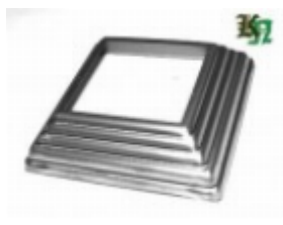
Основание блясины, арт. 13.360.01 108x108x1мм, кв.60x60мм Вес: 0.07 кг Цена: 40 руб.
