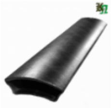
Поручень, арт. 12.033 3000x66x22мм Вес: 4.9 кг Цена (за штуку): 1 250 руб.
