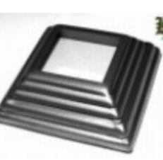
Основание баясины, арт. 13.319.01 80x80x1мм, кв.30x30мм Вес: 0.066 кг Цена: 26 руб.
