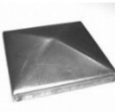
Заглушка на столб 80х80, арт. 15.056.36 80х80х1мм Вес: 0.08 кг Цена: 25 руб.
