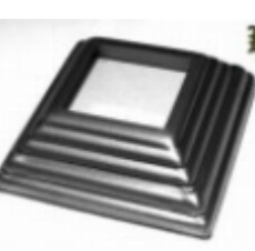
Основание баясины, арт. 13.321.01 90x90x1мм, кв.40x40мм Вес: 0.063 кг Цена: 29 руб.
