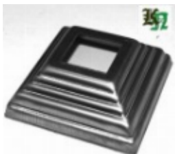
Основание баясины, арт. 10436.01 80x80x1мм, кв.25x25мм Вес: 0.075 кг Цена: 29 руб.
