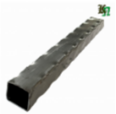
Труба профильная, арт. 60602Т 3000x60x60мм Вес: 9.8 кг Цена (за штуку): 1 200 руб.
