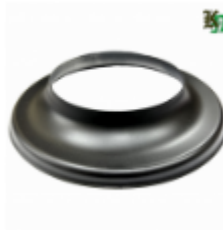
Переходник на трубу, арт. 8.270159 д=270мм, переход на д=159мм Вес: 0.6 кг Цена (за шт): 425 руб.
