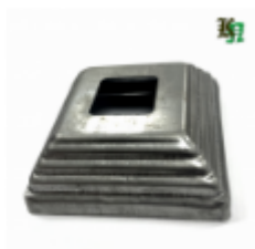
Основание баясины, арт. 10436.02 80x80x1мм, кв.25x25мм Вес: 0.075 кг Цена (за шт): 20 руб.
