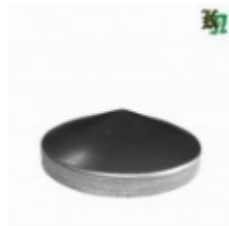
Заглушка, арт. 16.101.01 д=101x1мм Вес: 0.093 кг Цена: 53 руб.
