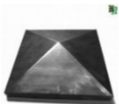
Заглушка на столб 120x120, арт. 15.058.02 120x120x1мм Вес: 0.142 кг Цена: 48 руб.
